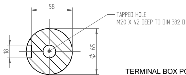
Przekrój A-A 1:2
